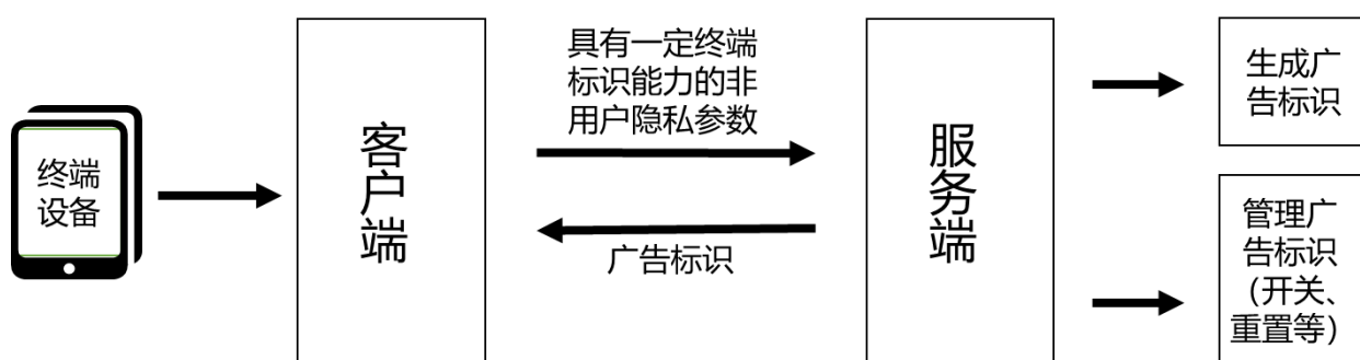
图1 技术框架
